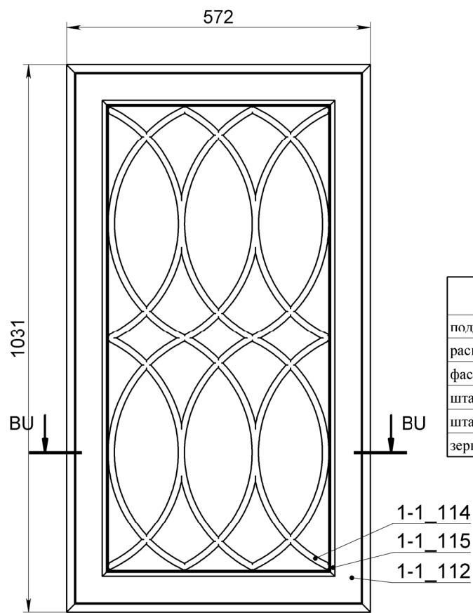
сборный фасад 1
